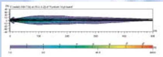
Lichtverdeling: Rally 3003 met High-Boost-reflector
